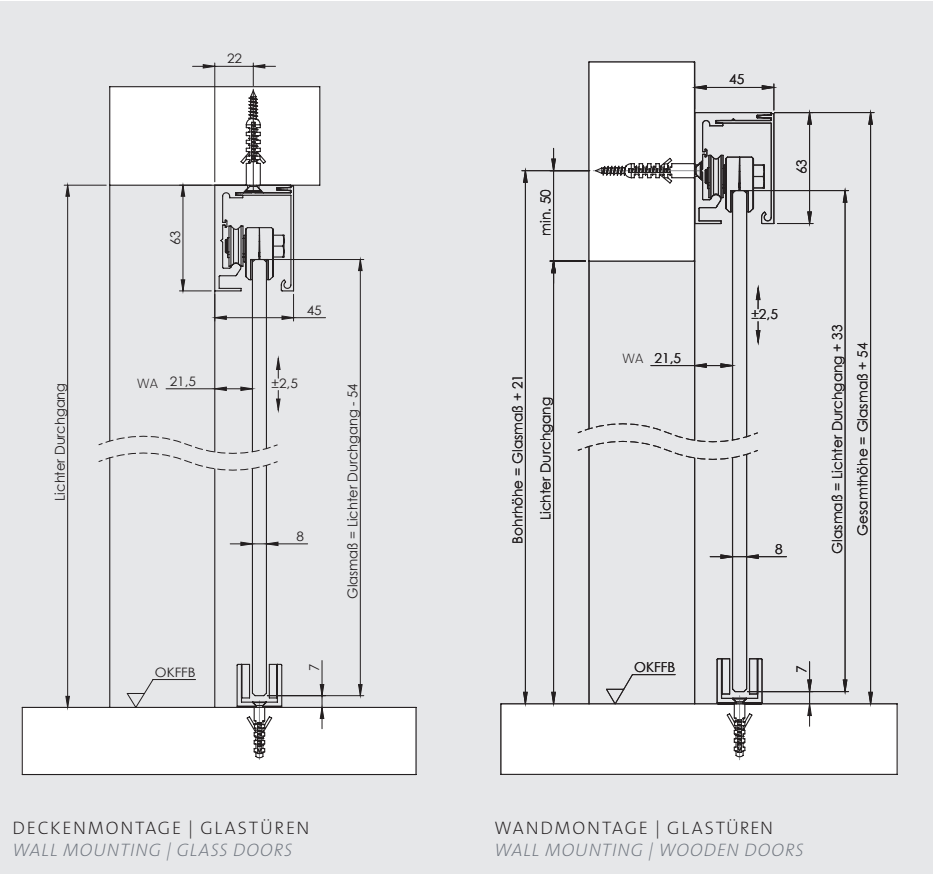
PLANE 120 DECKENMONTAGE FÜR RAUMHOHE LÖSUNGEN CEILING MOUNTING FOR FLOOR-TO-CEILING SOLUTIONS
